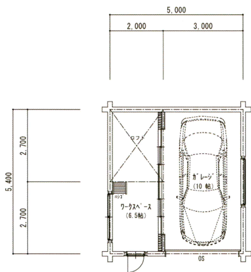
平面図
