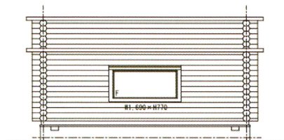
側面立面図
