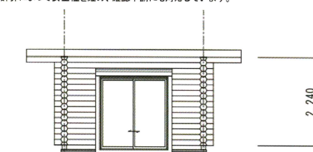
側面立面図
