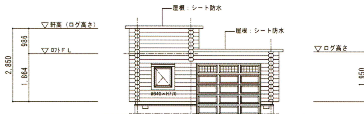
正面立面図
