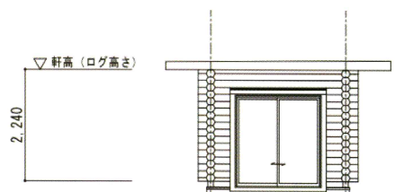
正面立面図
